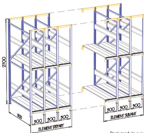
Rack module départ
